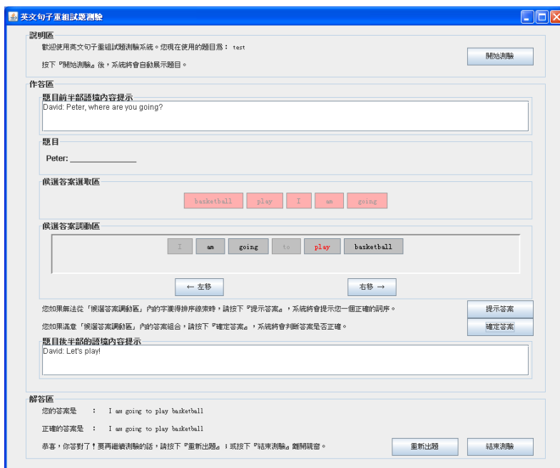
圖 11、練習介面
