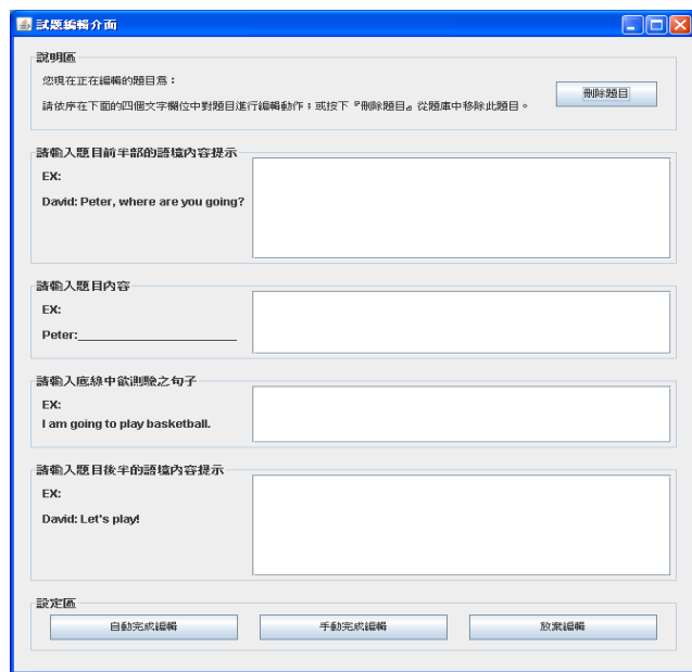
圖 9、編輯介面
