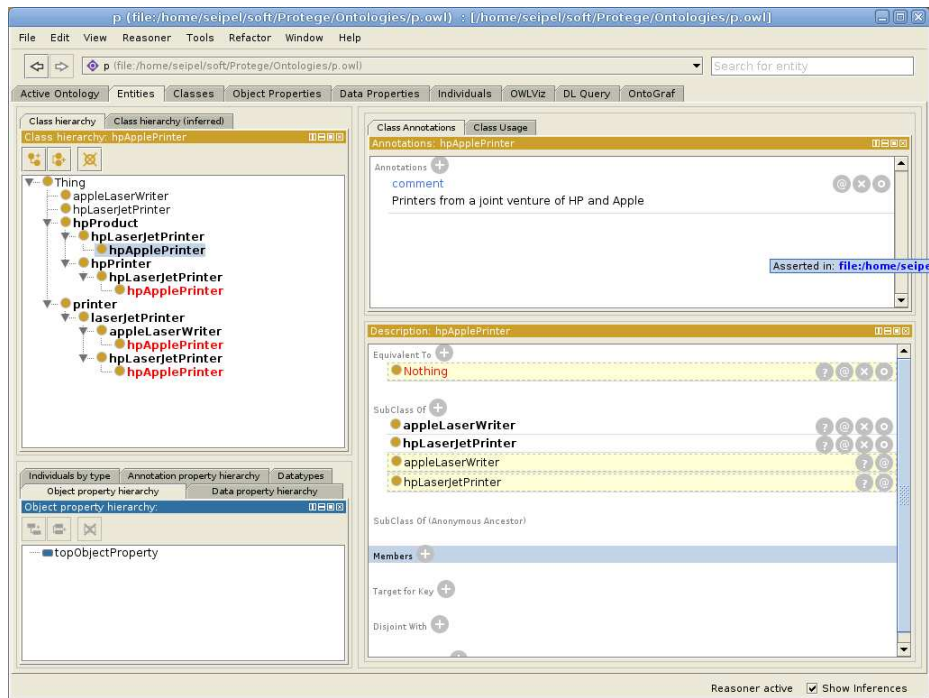
Fig. 1. The Printer Ontology in Protégé
