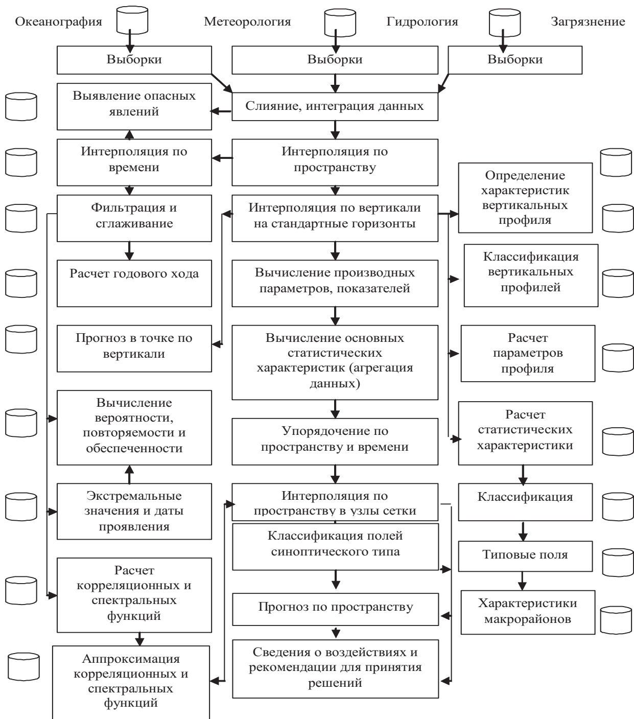
Рис. 1. Обобщенная блок-схема комплексной обработки гидрометеорологических данных [4]
