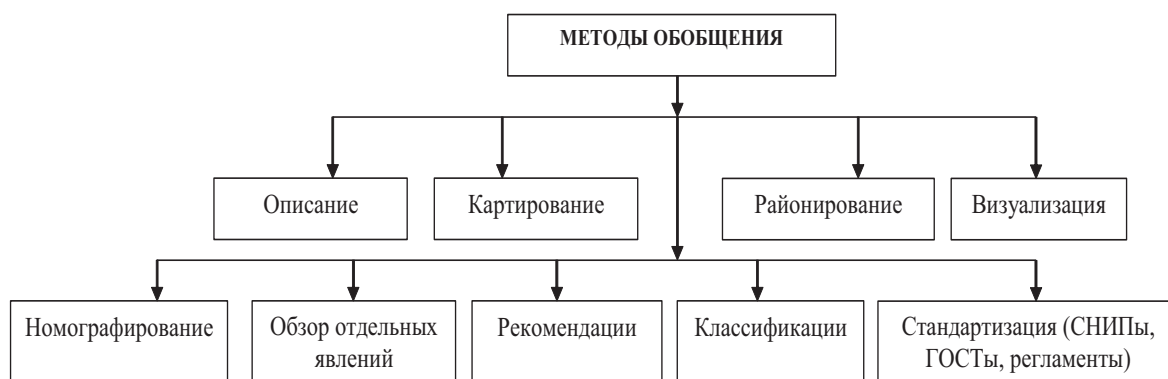
Рис. 4. Методы обобщения гидrometeorологической информации
