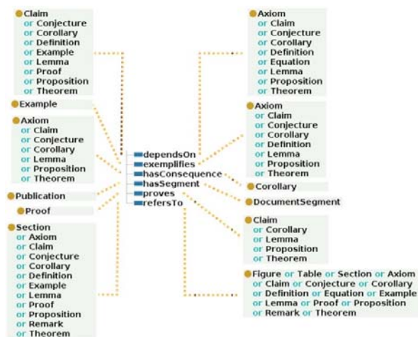
Рисунок 2 Элементы онтологии Mocassin [22]
