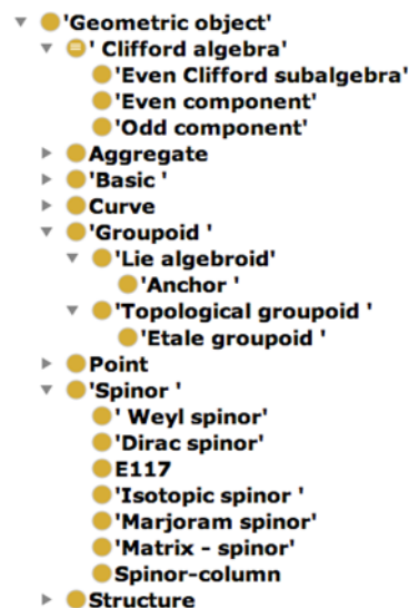
Рисунок 3 Фрагмент онтологии OntoMath PRO
