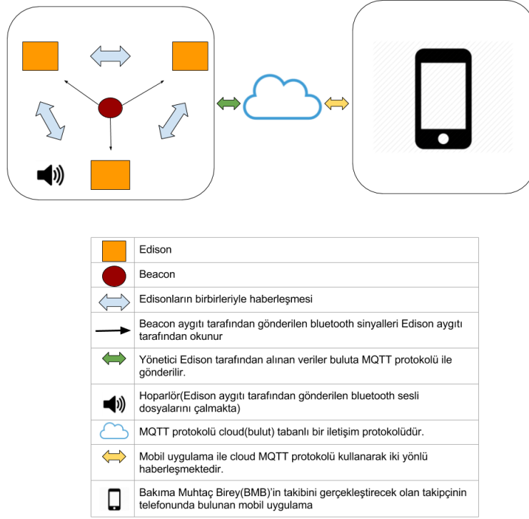
Şekil 1. Sistem Tasarımı
