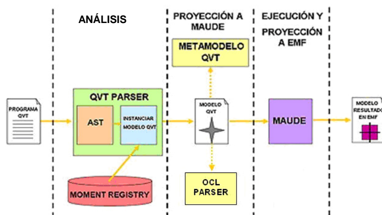
Figura 1. Proceso de ejecución de un programa QVT Relations en MOMENT
