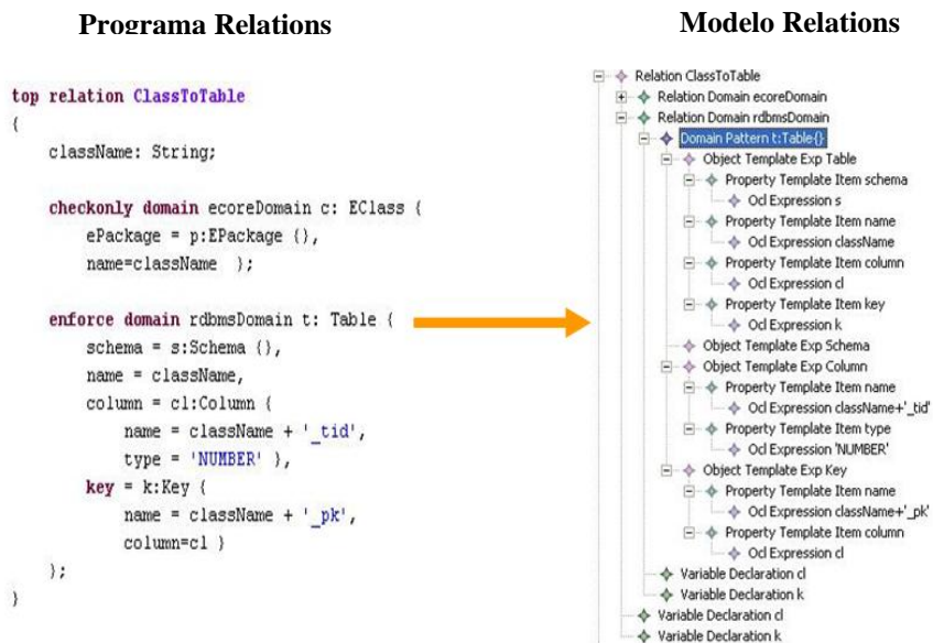
Figura 2. Vistas de programa Relations y modelo asociado.
