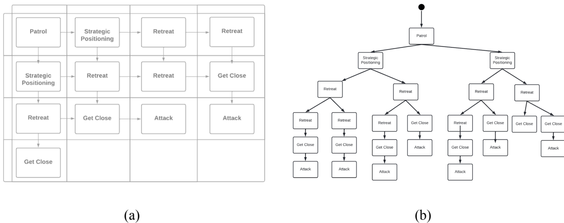
Figura 1: Matriz de comportamientos (a) y árbol de decisión del comportamiento del NPC (b).
