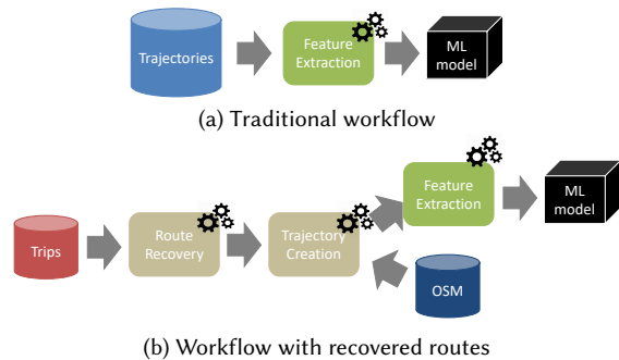
Figure 1: ETA prediction workflows
