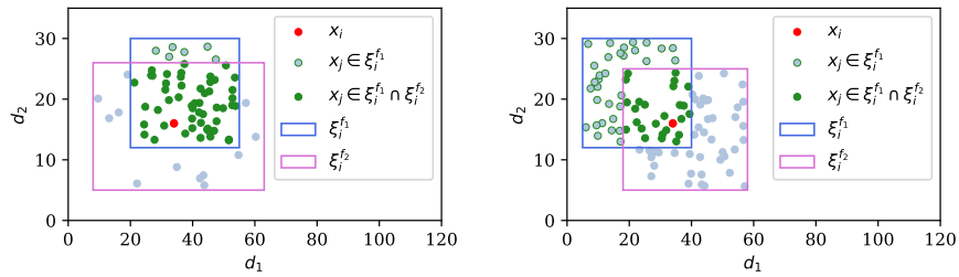
(d) Sensitive fragmentation ( \approx^S_C ).
