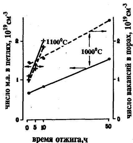
Рис.2. Изменение числа междоузельных атомов в дислокационных петлях и вакансий в гелиевых порах в Мо в зависимости от времени послерадиационного отжига при 1000 и 1100°C.
