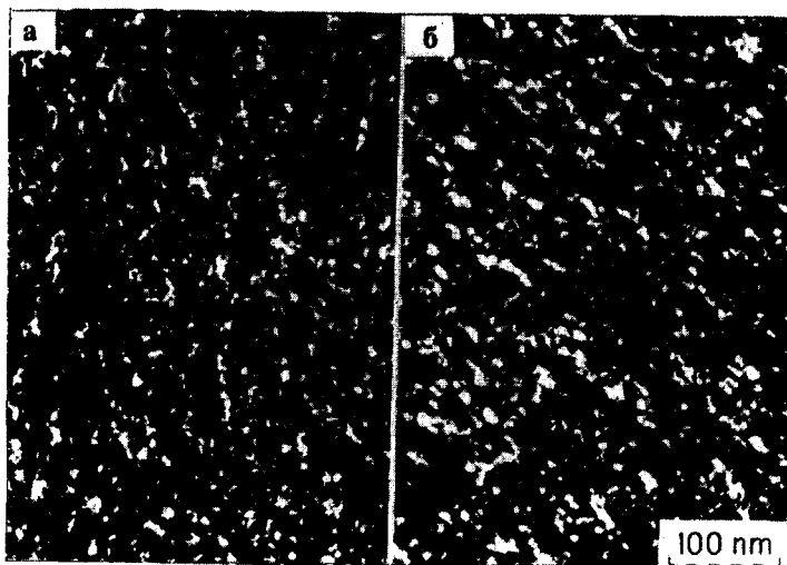
Рис.6. Дефектная структура в Мо после облучения при 60 0 С. а - нейтронами деления ( 7 \times 10^{-2} сна), б - альфа-частицами с энергией 50МэВ ( 7 \times 10^{-2} сна)
