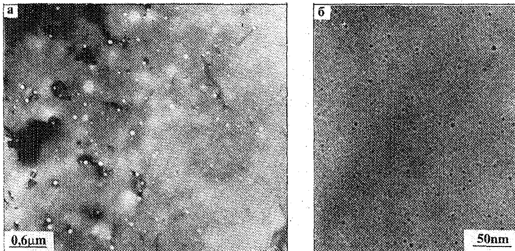
Рис.5. Развитие гелиевых пор в Ni ( 2 \times 10^{-2} ат.%He) в результате отжига при 800^{\circ}\text{C} : а - в обедненной от дислокационных петель приграничной области А (см.рис.4), б - в теле зерна (область В, см. рис.4)
