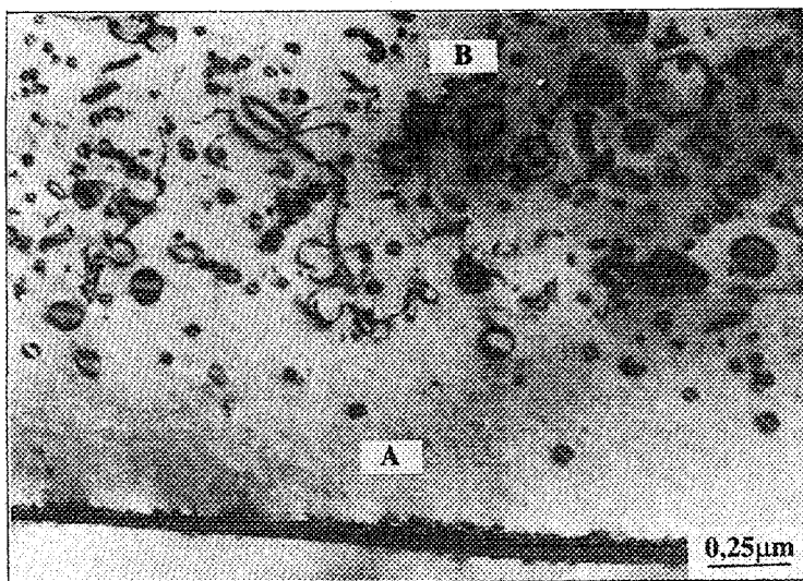
Рис.4. Дислокационные петли в Ni, легированном гелием до 2 \times 10^{-2} ат.% и отожженном при 600^\circ\text{C} в течение 1 ч
