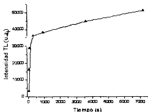
Figura 2. Respuesta TL de películas delgadas de óxido de aluminio como función del tiempo de irradiación con UV.
