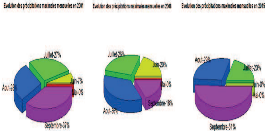
Figure 7 : Répartition des précipitations maximales mensuelles par septennat de 2001 à 2015
