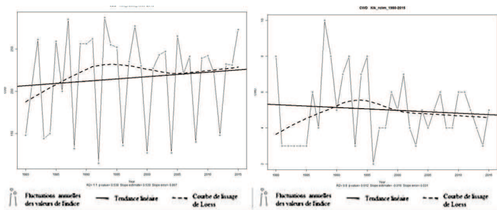
Figure 3 : Evolution annuelle et tendance linéaire des valeurs des indices climatiques (CDD et CWD)
