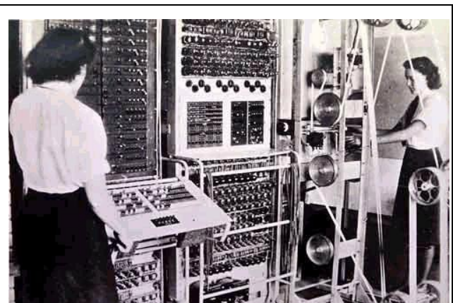
Il Colossus Mark II. Il pannello di controllo a sinistra viene utilizzato per regolare i settaggi del decodificatore di Lorenz. I nastri con i dati sono a destra
