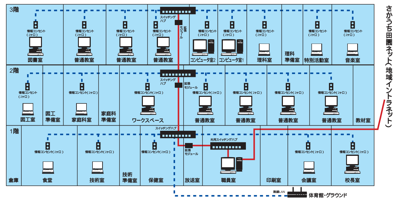
坂内村立坂内小中学校LAN系統図
