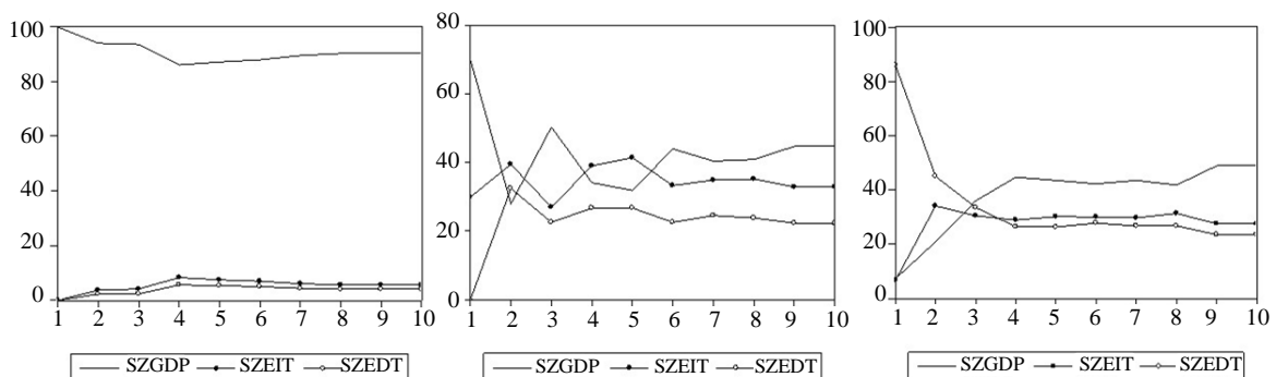
Figure 3. Variance decomposition of SZGDP, SZEIT, SZEDT.
