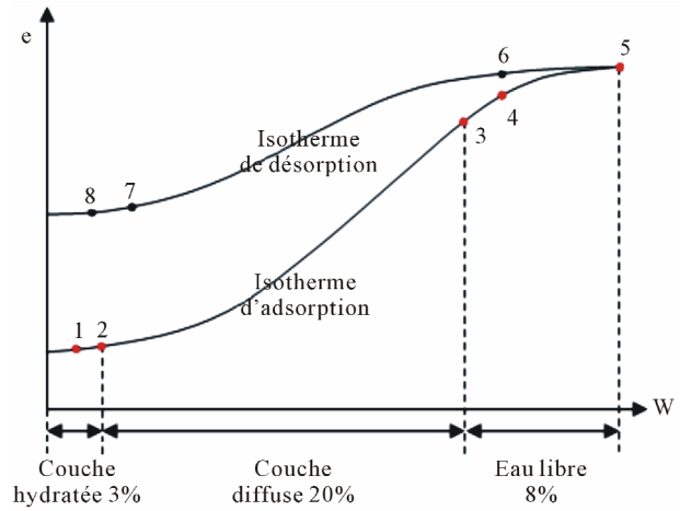
1: liaisons de Van der Waals, de cimentation, de cristallisation et de condensation; 2: liaisons colloïdale, intermoléculaire et de coagulation (les phases 1 et 2 constituent l'étape de destruction des liaisons structurales); 3: fin de la formation de la couche diffuse; 4: fin de remplissage des pores interparticulaire; 5: fin d'adsorption, limite de gonflement; 6: sortie de l'eau libre, entrée de l'air dans les macropores; 7: formation des liaisons structurales entre les particules, entrée d'air dans les micropores; 8: limite de retrait.
