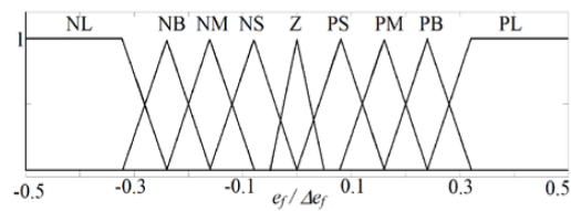
(a). MFs of FLC f input
