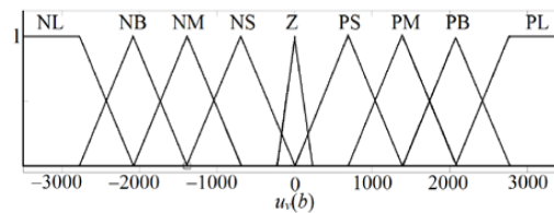
(d). MFs of FLC v output
