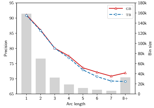
(b) Precision
