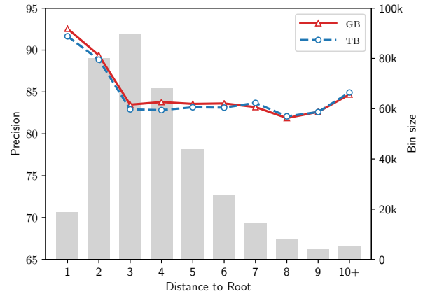
(b) Precision
