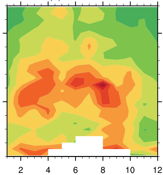
(d) MISR AOD
