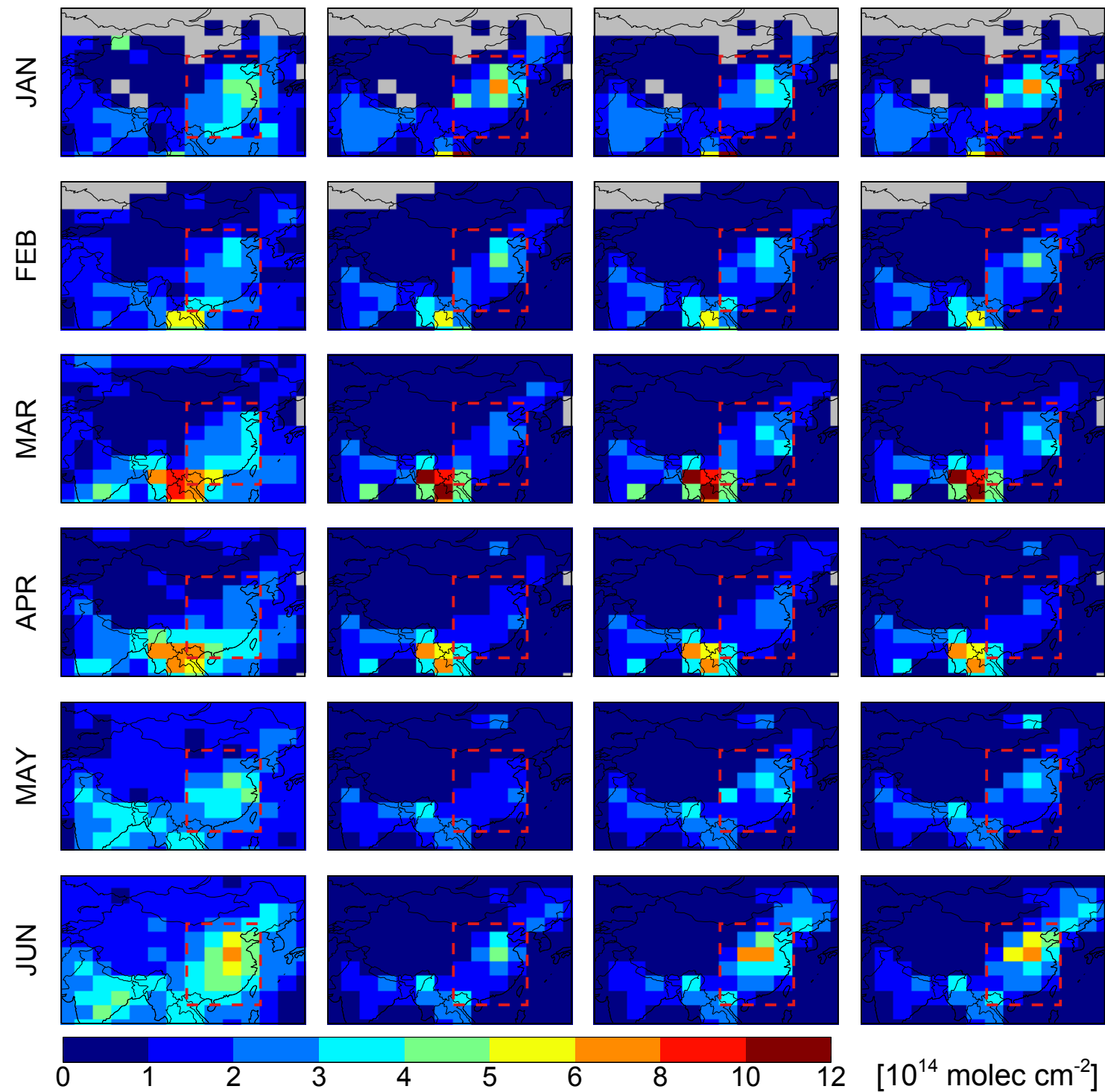
(a) GOME-2A
