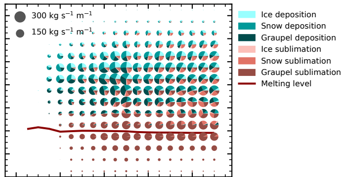
(d) THOM 2500 cm -3
