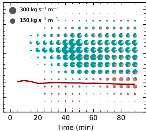
(d) THOM 2500 cm -3
