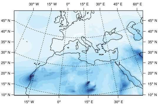
MODIS Terra
