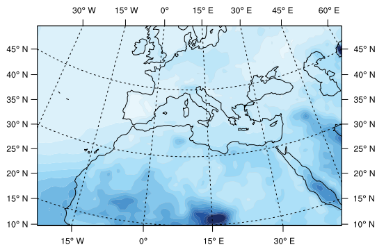
MODIS Aqua
