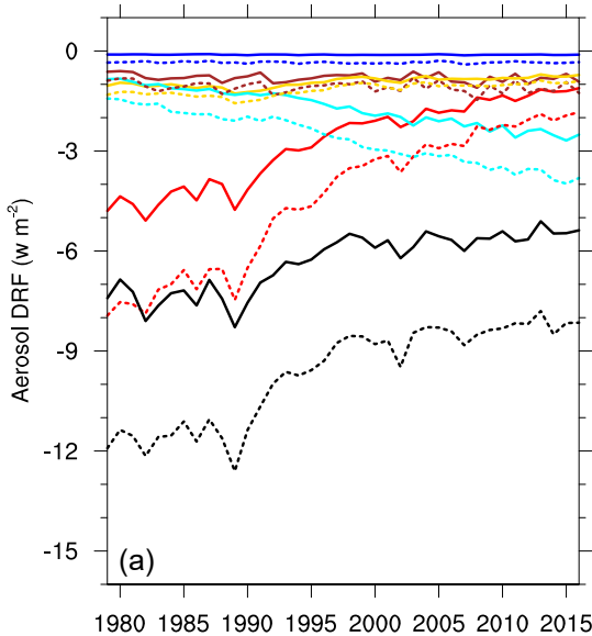
Europe (TOA)
