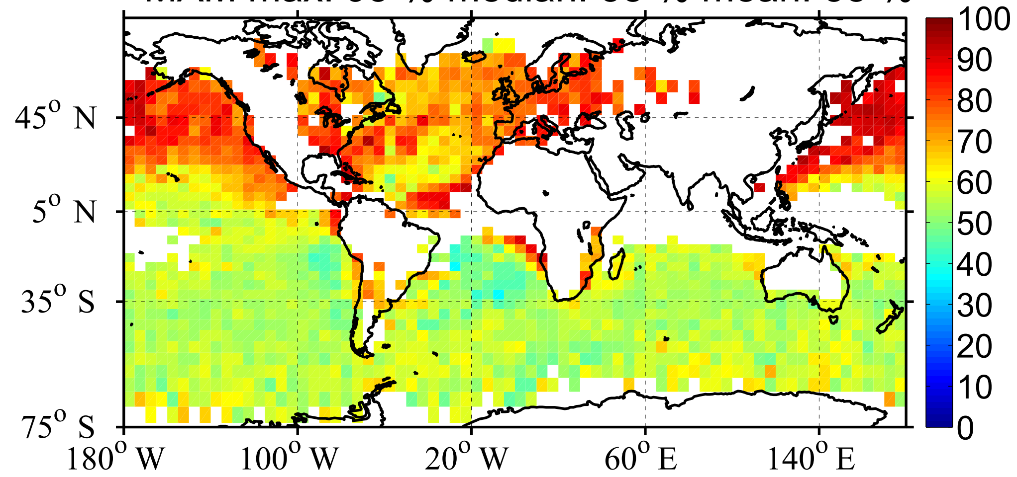
MAM max: 95 % median: 58 % mean: 58 %
