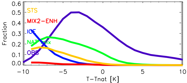
CALIOP V2
