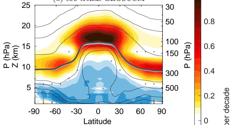
(b) e90 trends GEOSCCM
