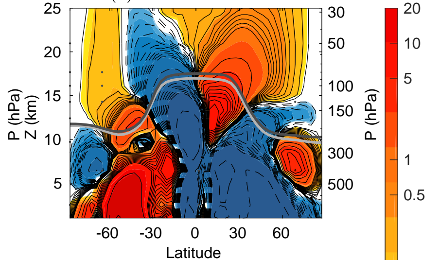
(d) \Psi^* trends GEOSCCM
