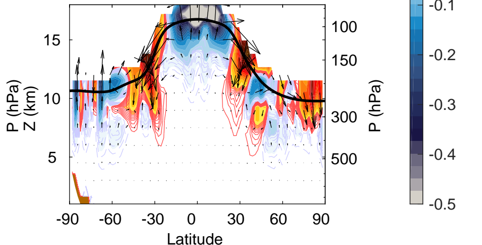
(d) st80 ADV trend WACCM
