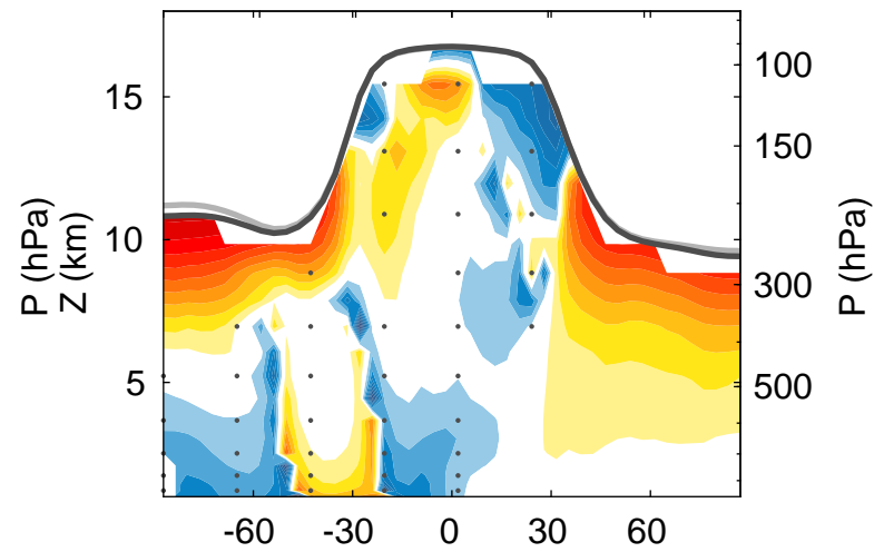
(d) st80 trends WACCM fGHG
