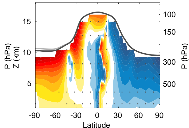
(d) st80 trends WACCM fGHG
