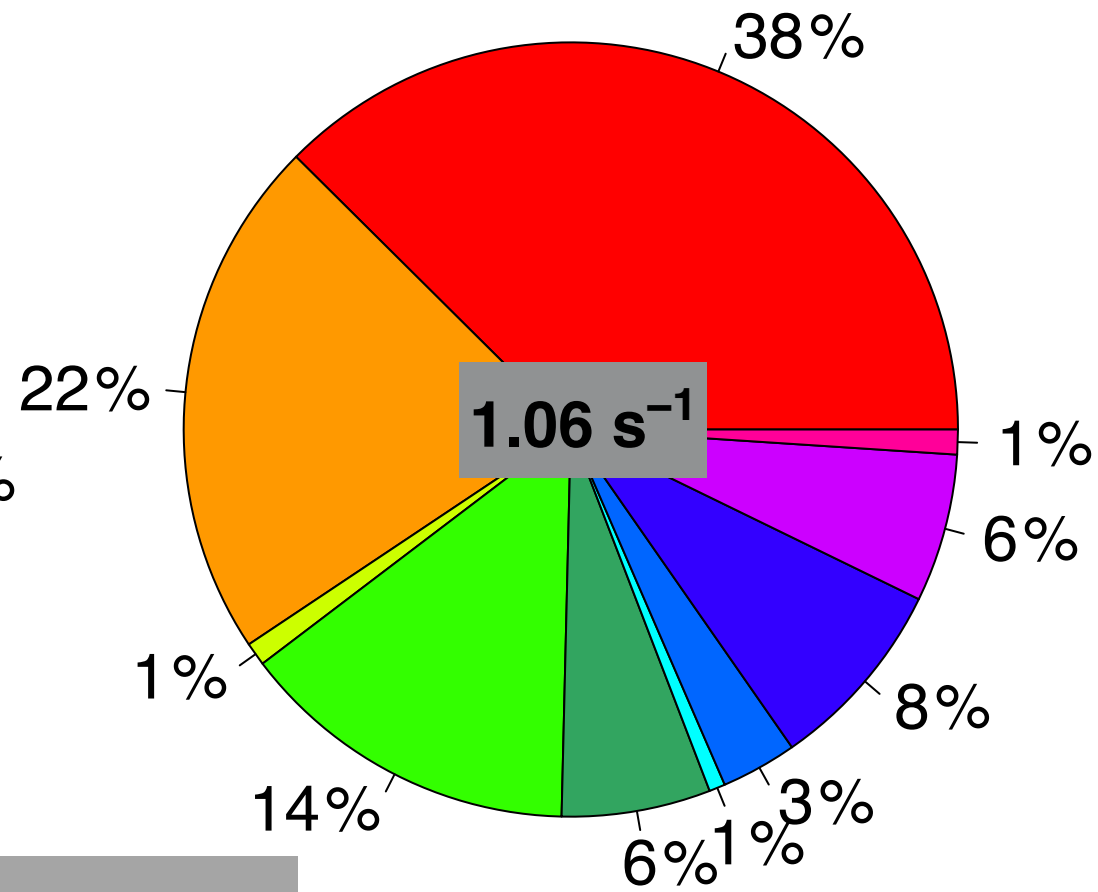
Model (NH)
