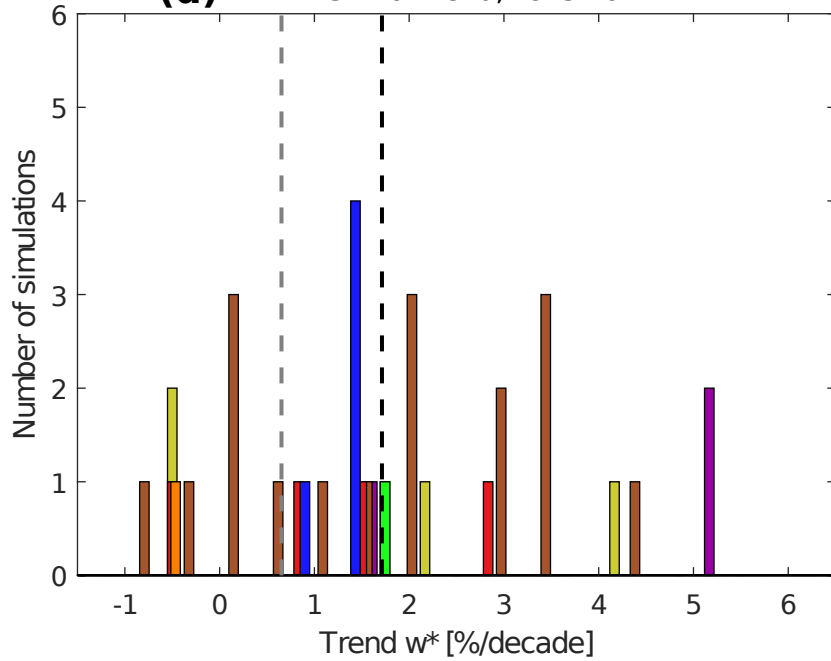
(d) w^* 1.5 hPa Trend, 1975-2014
