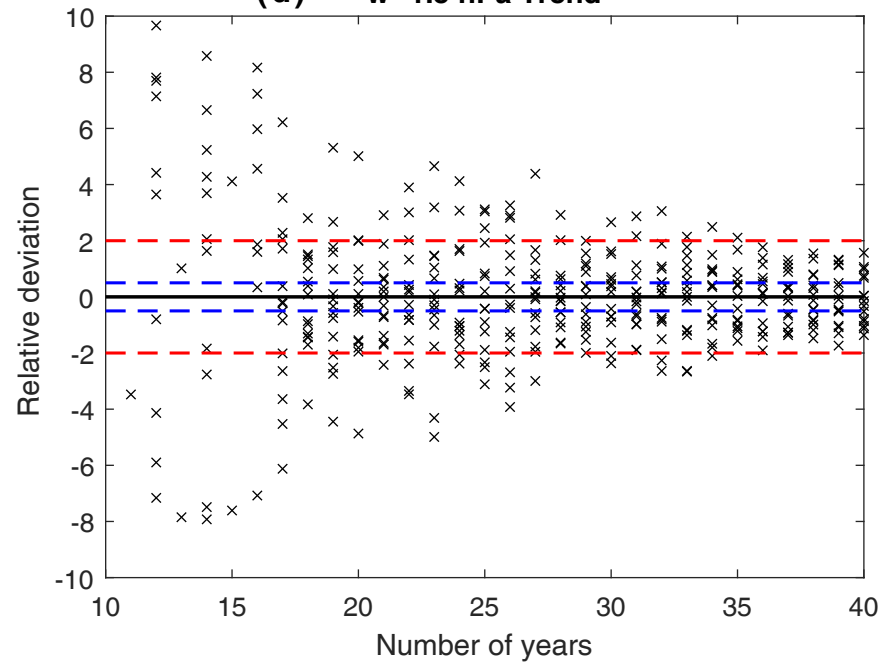
(d) w^* 1.5 hPa Trend
