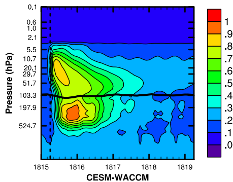
CESM-WACCM
