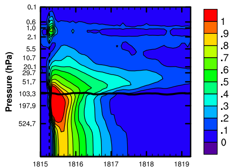
LMDZ-S3A band
