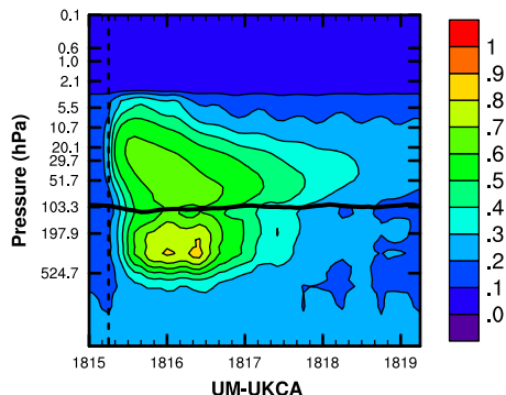
UM-UKCA
