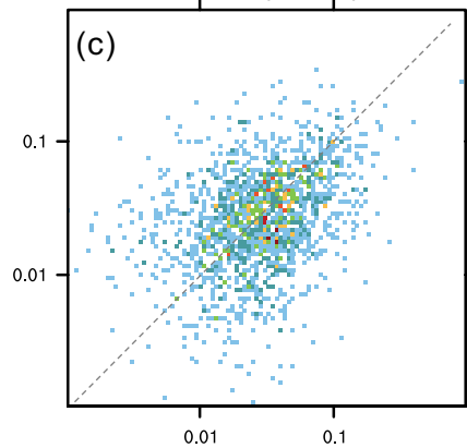
AERONET cmAOD
