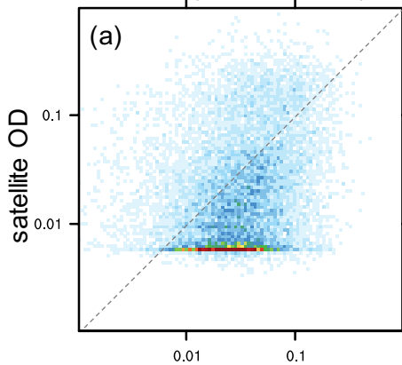
AERONET cmAOD
