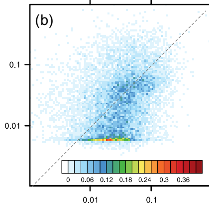
AERONET cmAOD
