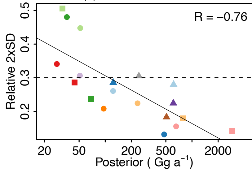
(d) Posterior emissions
