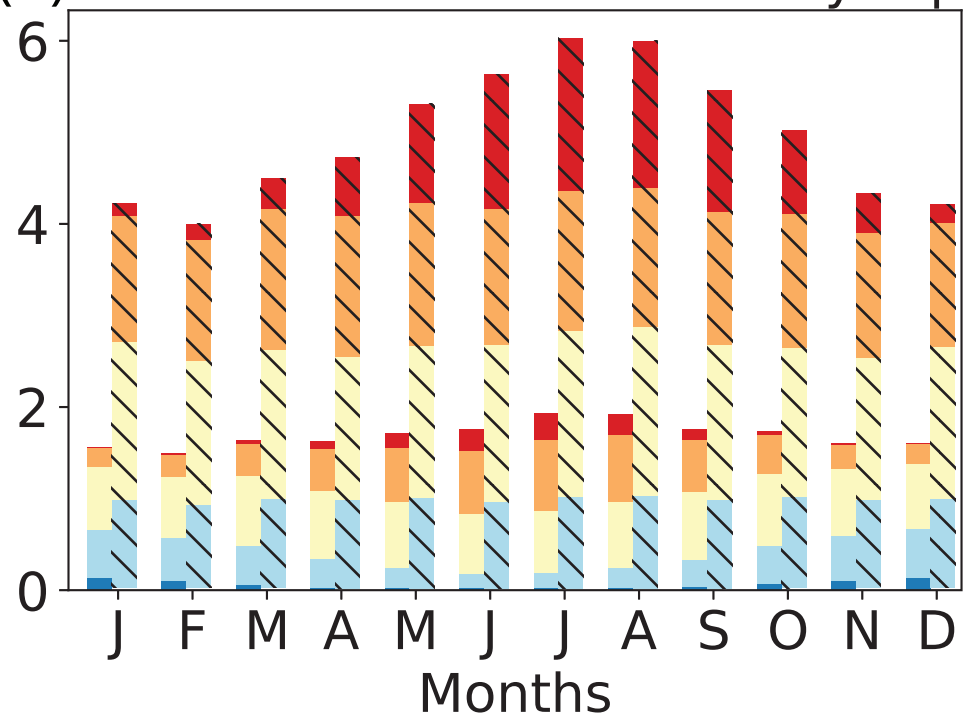
(d) 2016 ChemLoss DryDep
