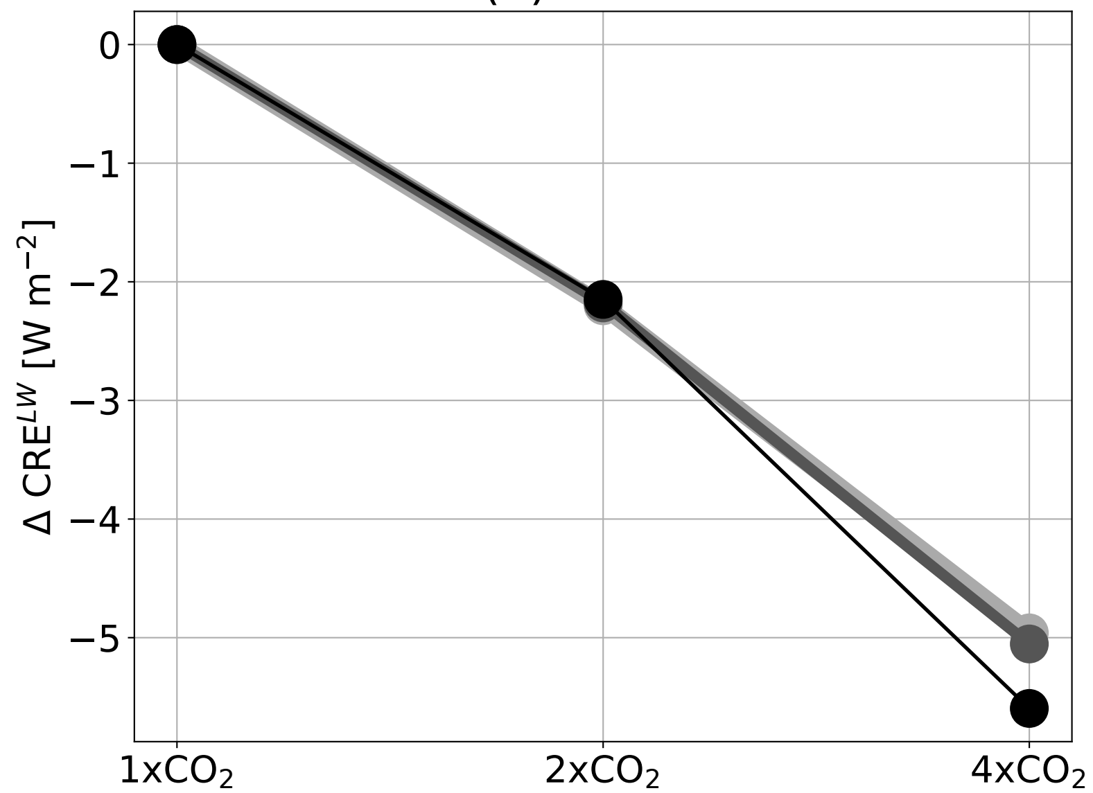
(d) \text{CRE}^{LW}
