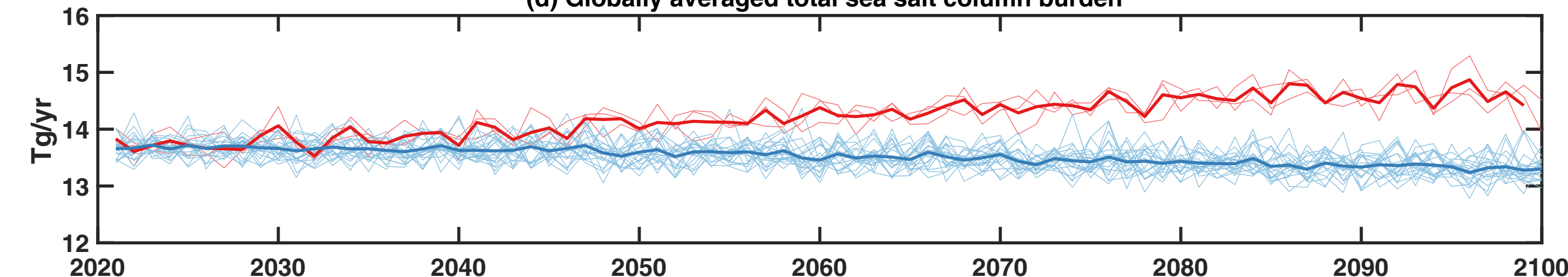
(d) Globally averaged total sea salt column burden
