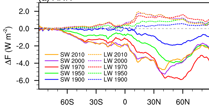
(a) ANN
