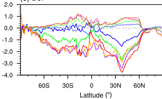
(e) DJF
