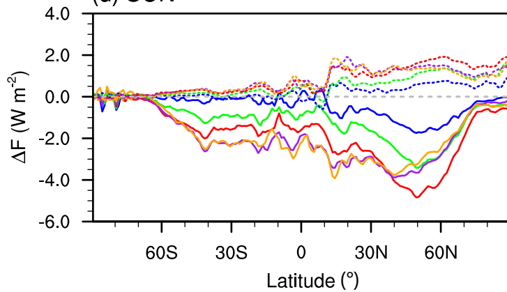
(d) SON
