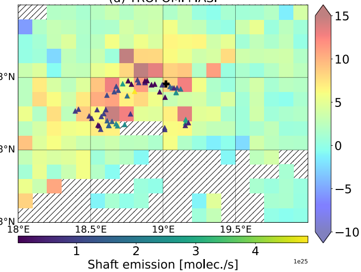
(d) TROPOMI+IASI
