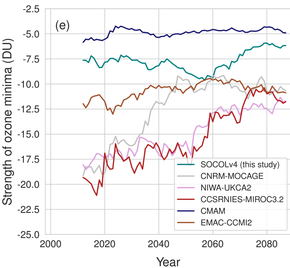
SSP2-4.5 - CCMI-2022
