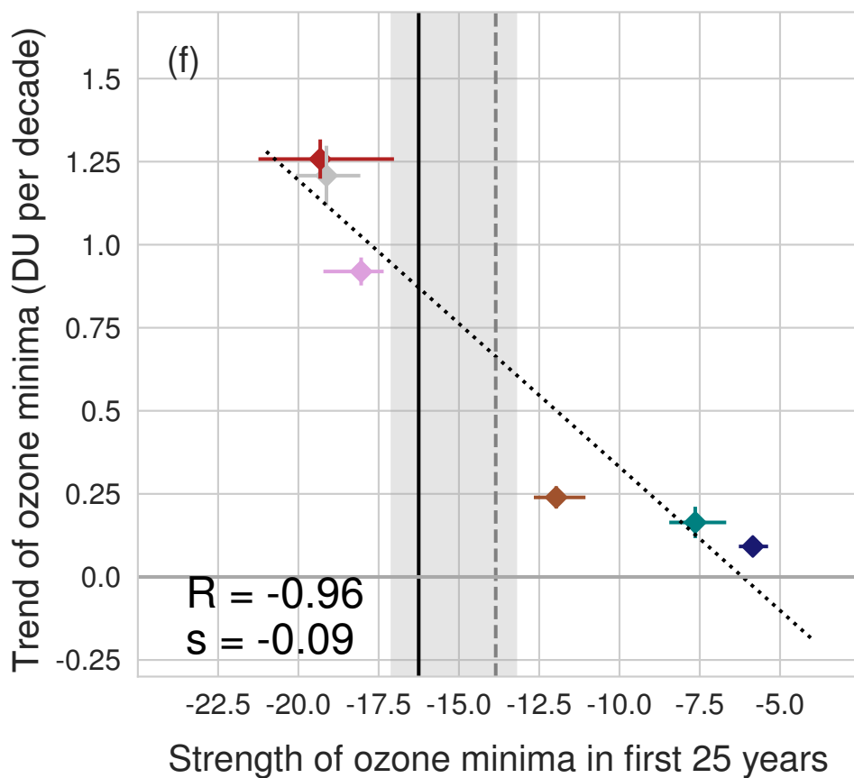
SSP2-4.5 - CCMI-2022
