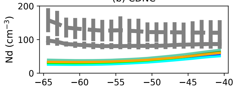
(b) CDNC
