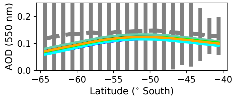
(f) AOD
