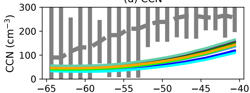
(d) CCN
