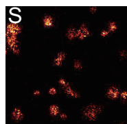
(d) 9 Aug 01:22 (smoke and cloud)
