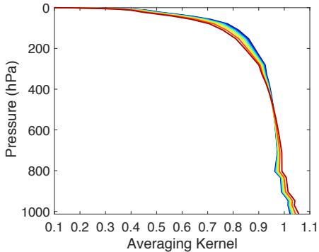
(b) CH 4
