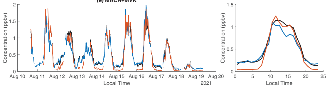
(e) MACR+MVK
