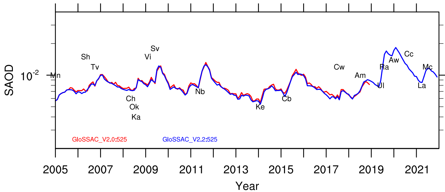
525 nm Global SAOD
