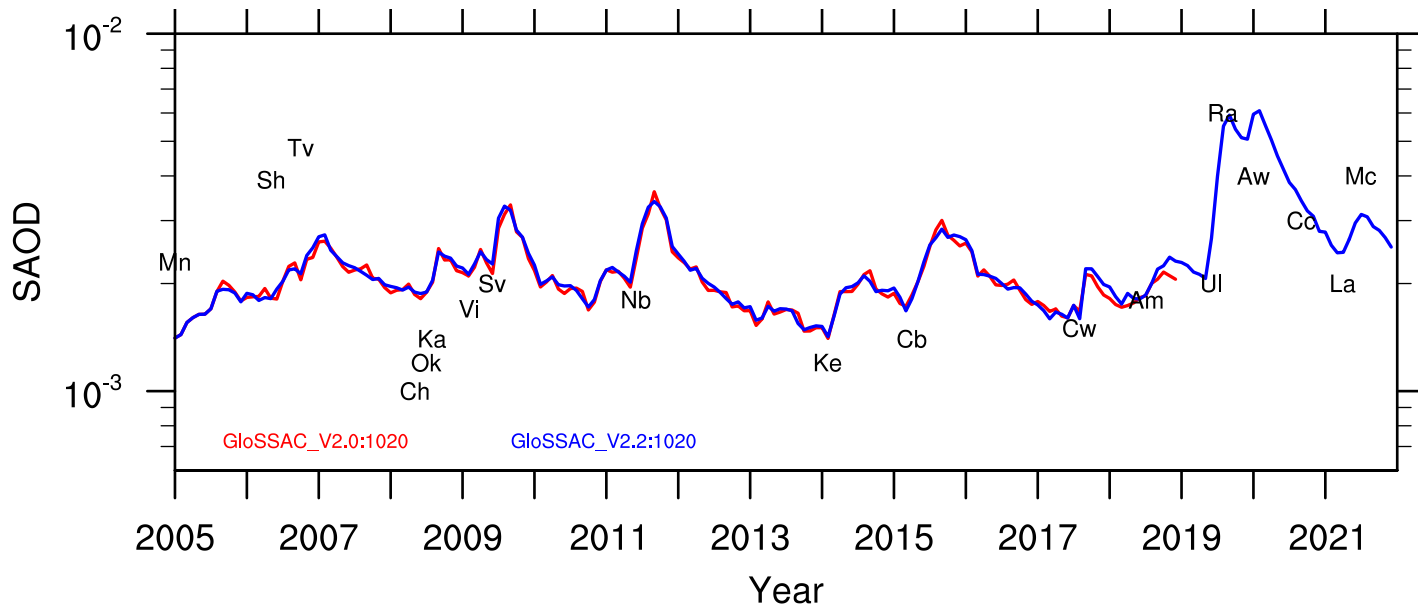
1020 nm Global SAOD
