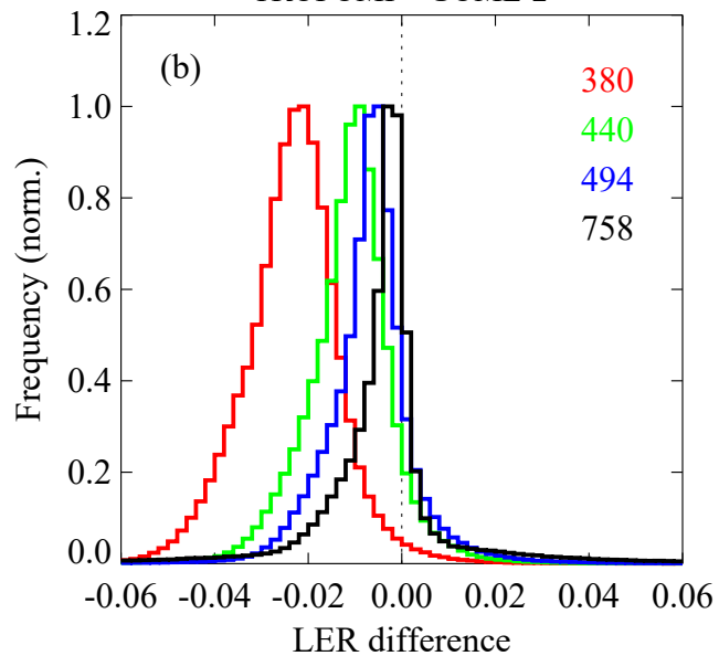
TROPOMI - OMI
