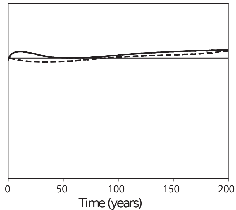
UVic ESCM 2.10
