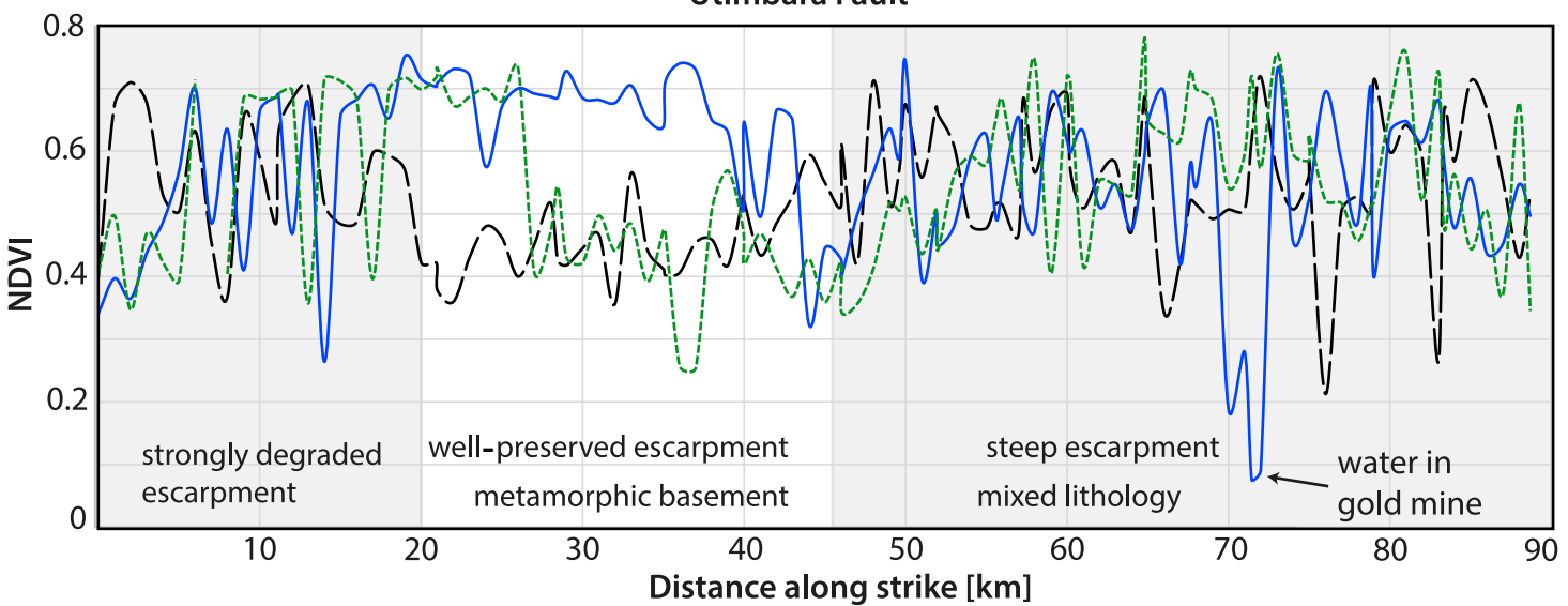
Utimbara Fault
