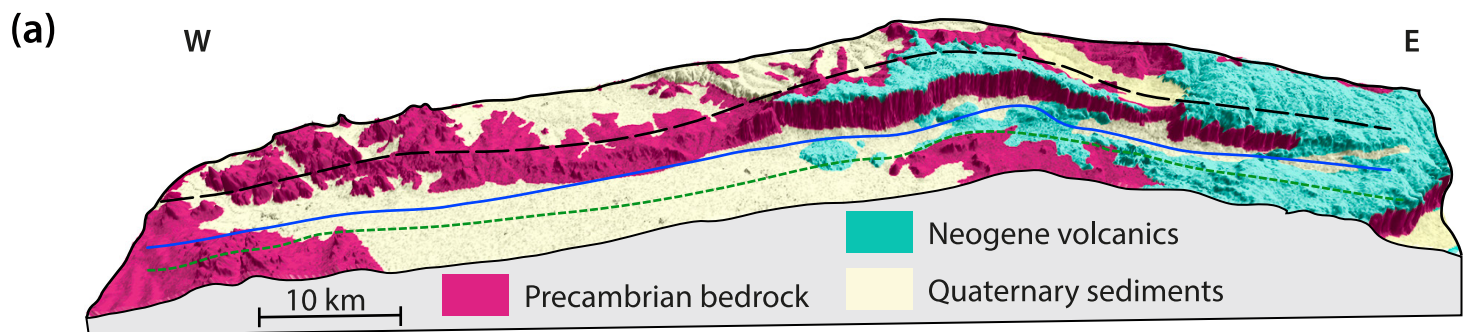
Utimbara Fault
