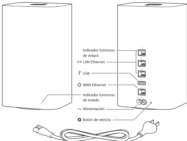
Cable de alimentación (Su cable de alimentación puede ser distinto.)
